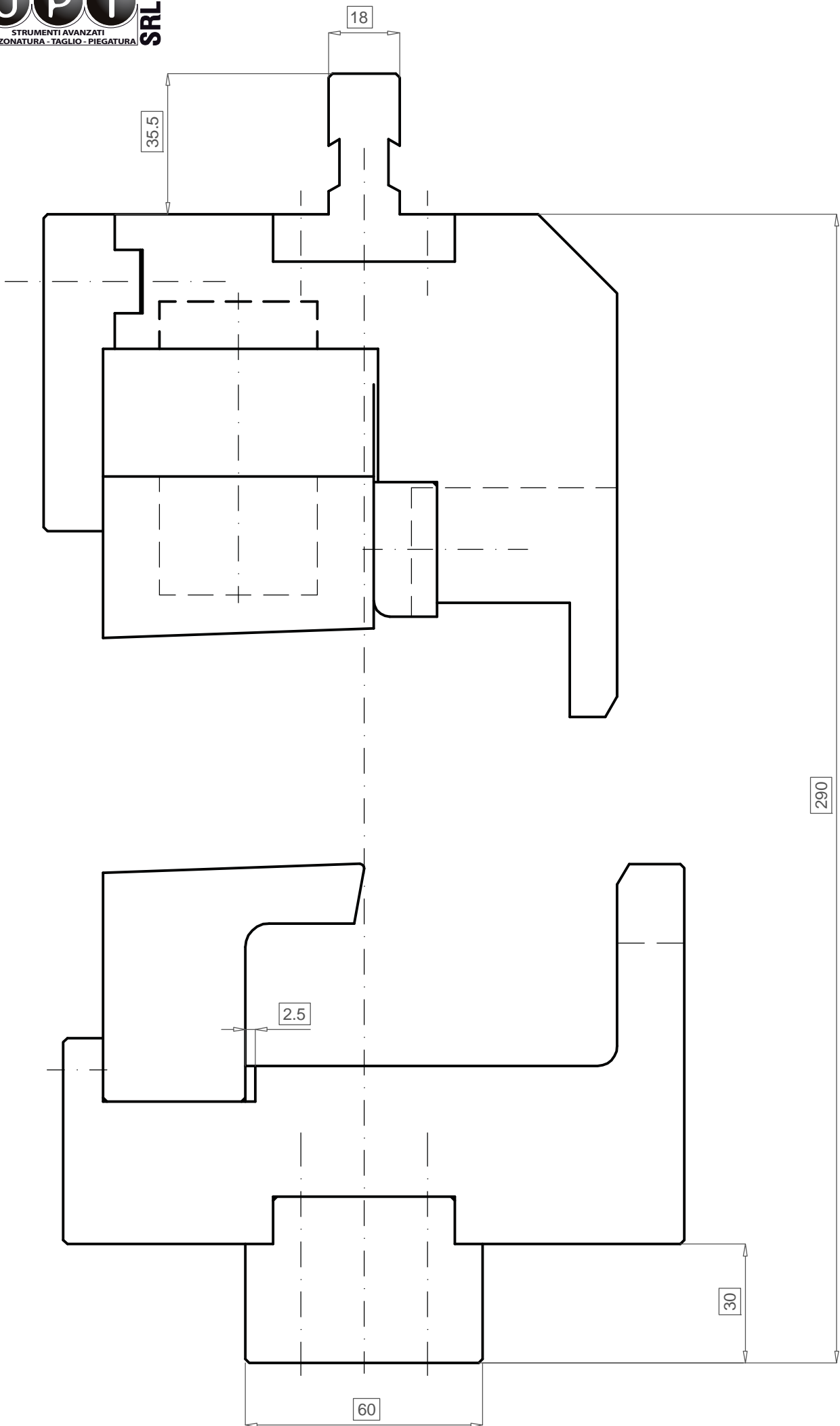
STAMPO TANGENZIALE APERTO
